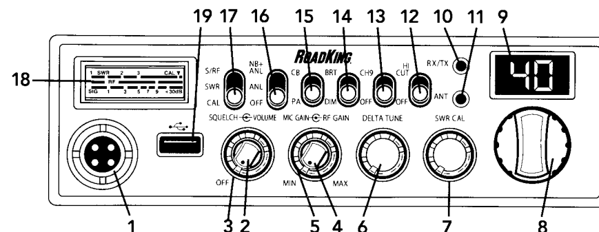
VUE DE FACE - PANNEAU RETRO-ÉCLAIRÉ DE LA RADIO RK5640
